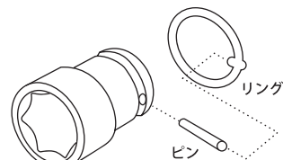
インパクトレンチ用ソケット
