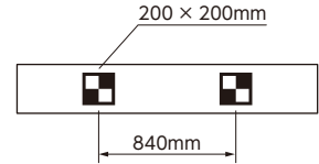
MAGNET TARGET SHEET (MITSUBISHI1) No.AT120-051
