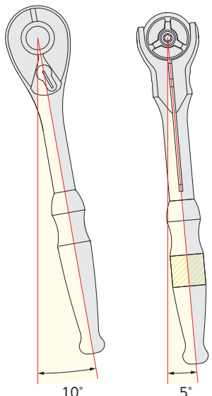
スタンダード ラチェットハンドル (BR3E)
